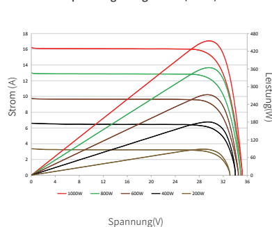
Strom-Spannungs- und Leistungs-Spannungs-Diagramme(445W)
